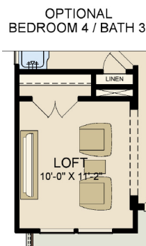
OPTIONAL LOFT
